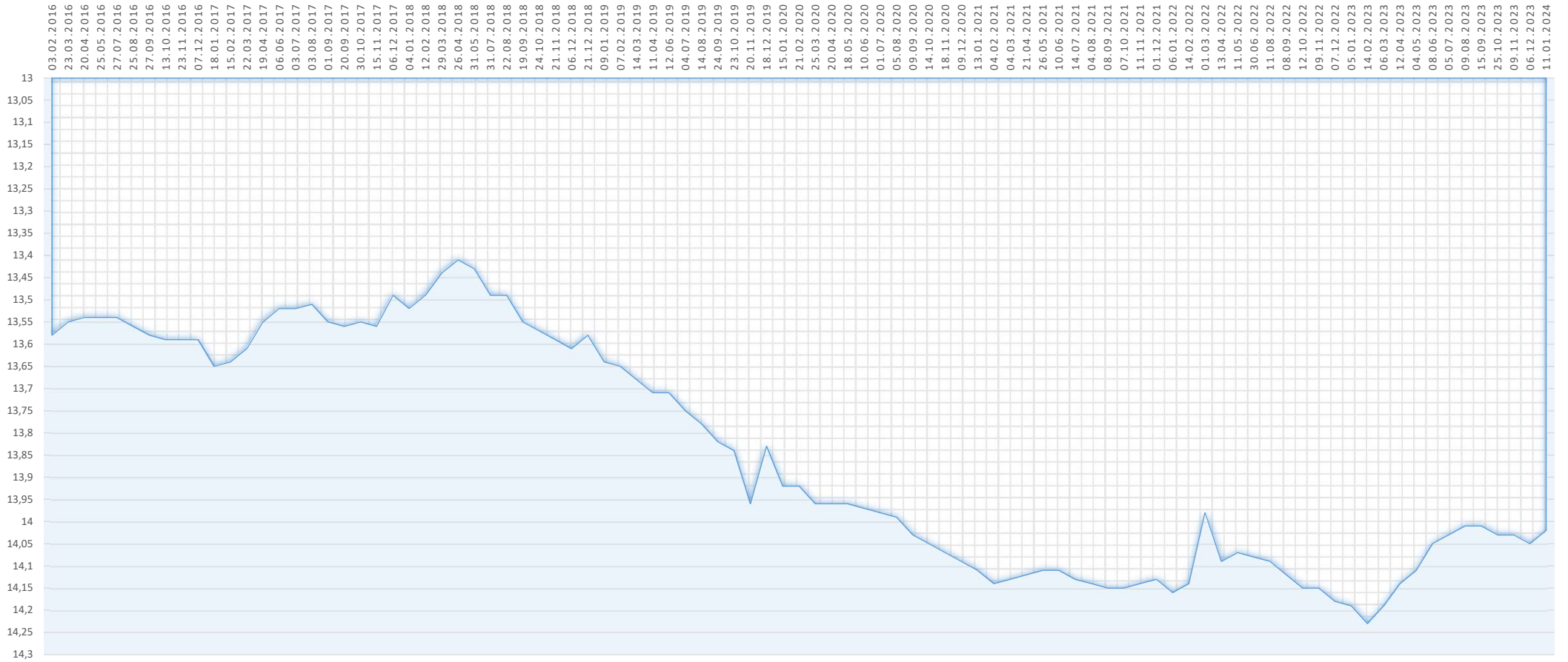
Grundwasserpegel 09/15 Wasserstand unter Messpunkt [m]
